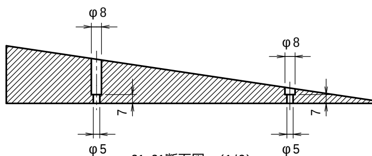
S1-S1断面図 (1/3)
